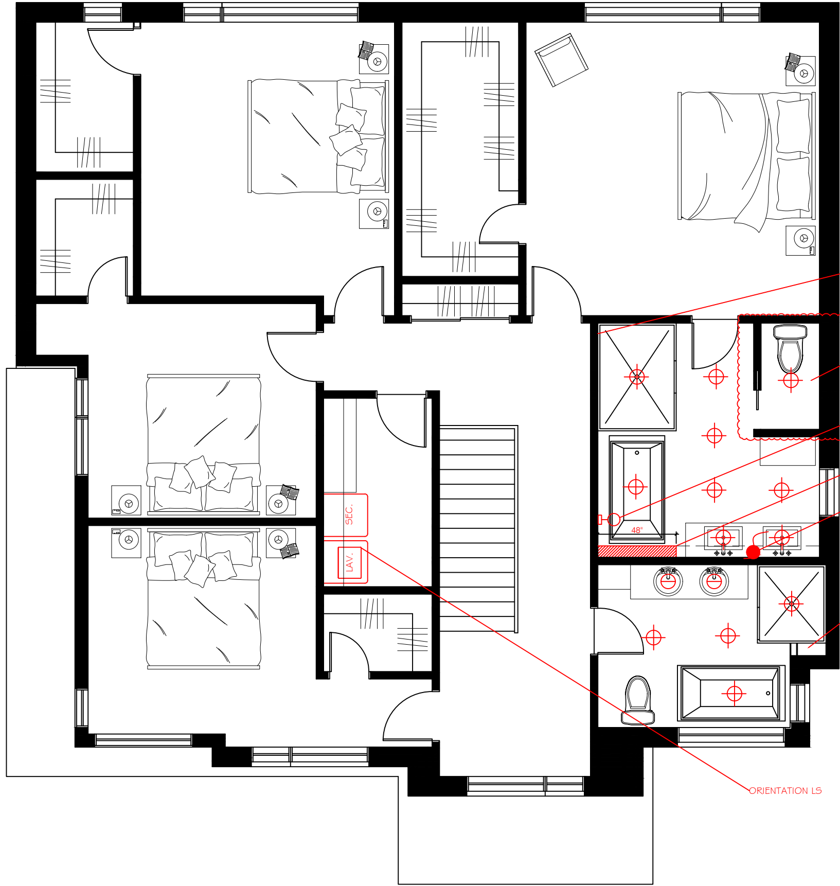
1 PLAN ÉTAGE - CONSTRUCTION D2 ÉCHELLE: 3/16" = 1'-0"
